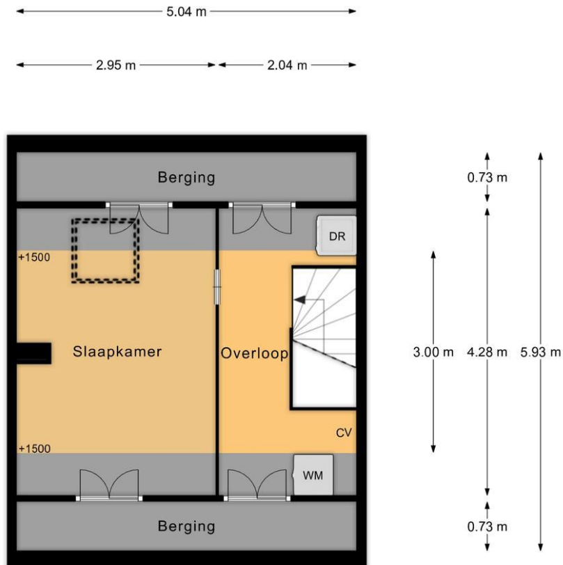
2e verdieping
