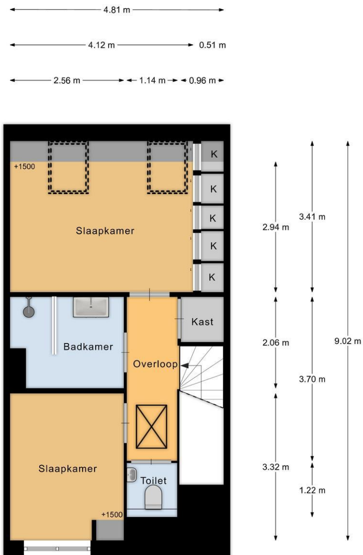
2e verdieping
